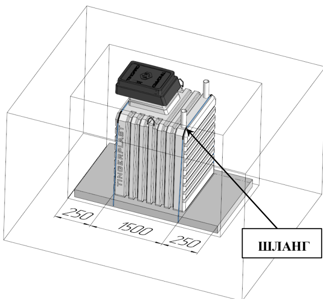
Рисунок 4 – Установка погреба
