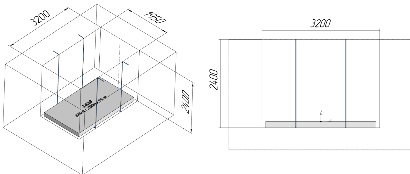
Рисунок 1 – Размеры котлована под установку плиты
