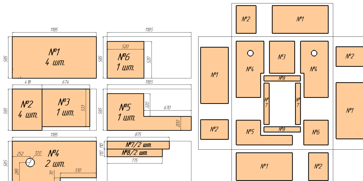
Рисунок 7 – Карта раскроя утеплителя
