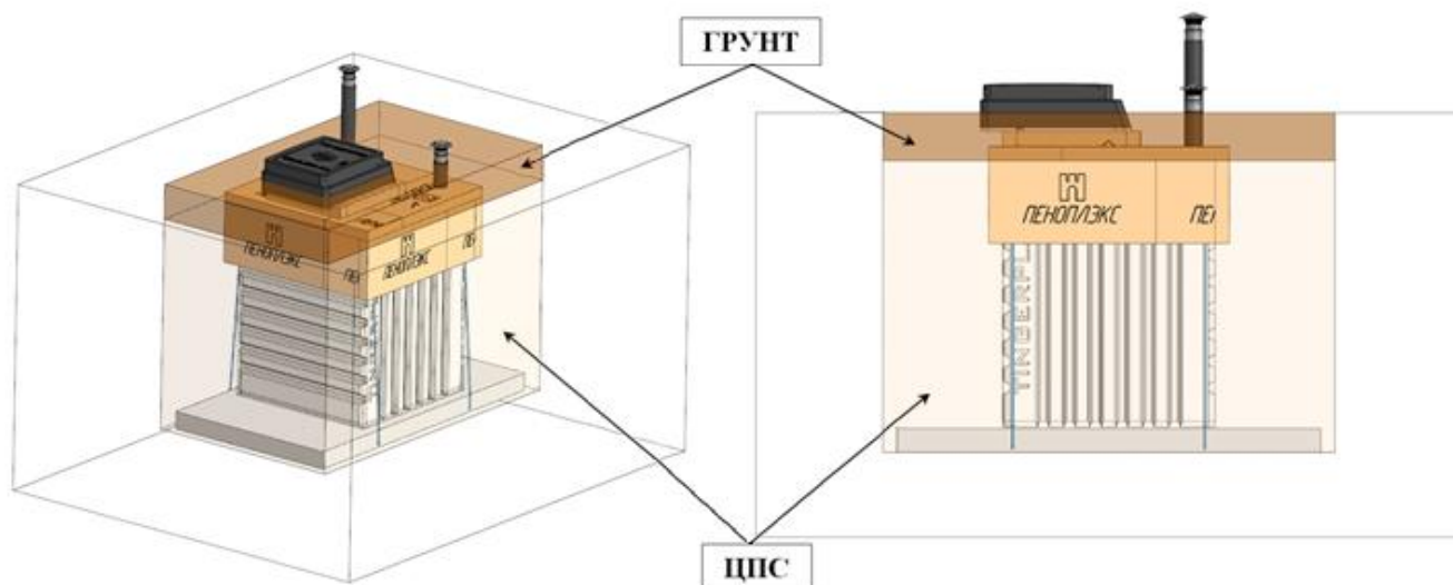
Рисунок 10 – Засыпка погреба
