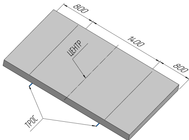
Рисунок 2 – Закладка тросов
