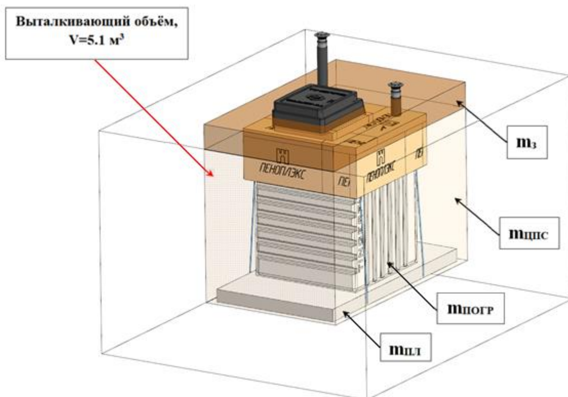
Рисунок 10 – Расчет якорения погреба
