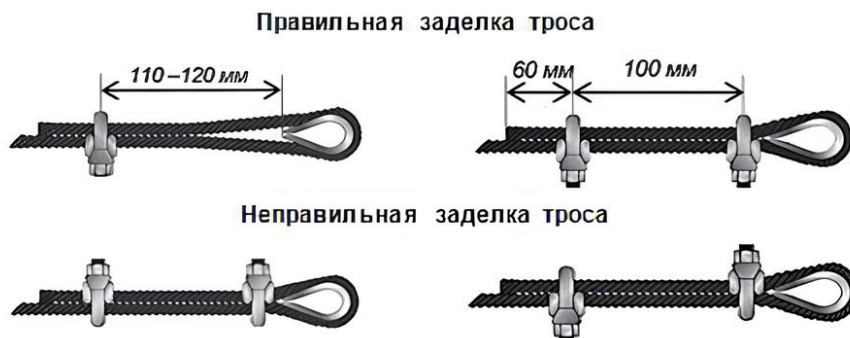
Рисунок 6 – Заделка троса
