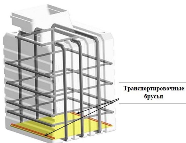
Рисунок 9 – Транспортировочные брусья на полу
